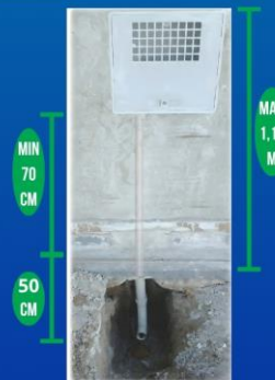
VISÃO FRONTAL DA CAIXA INSTALADA
