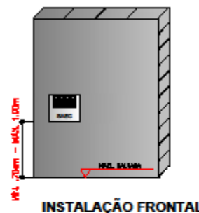
INSTALAÇÃO FRONTAL
