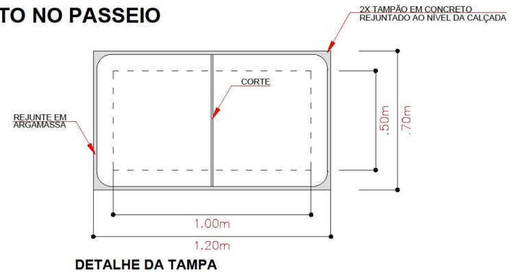
DETALHE DA TAMPA
