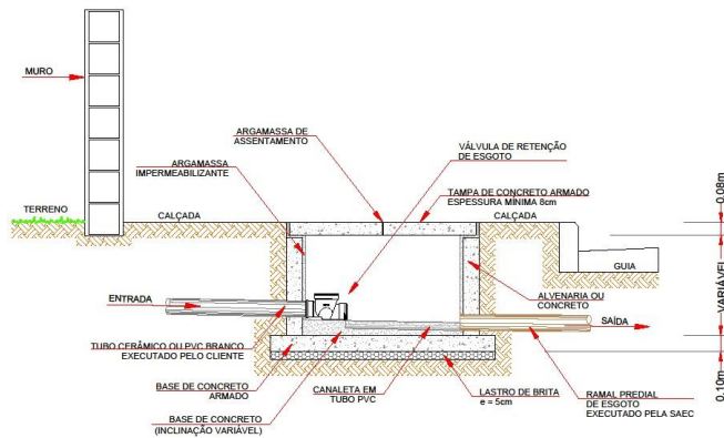
CORTE AA
